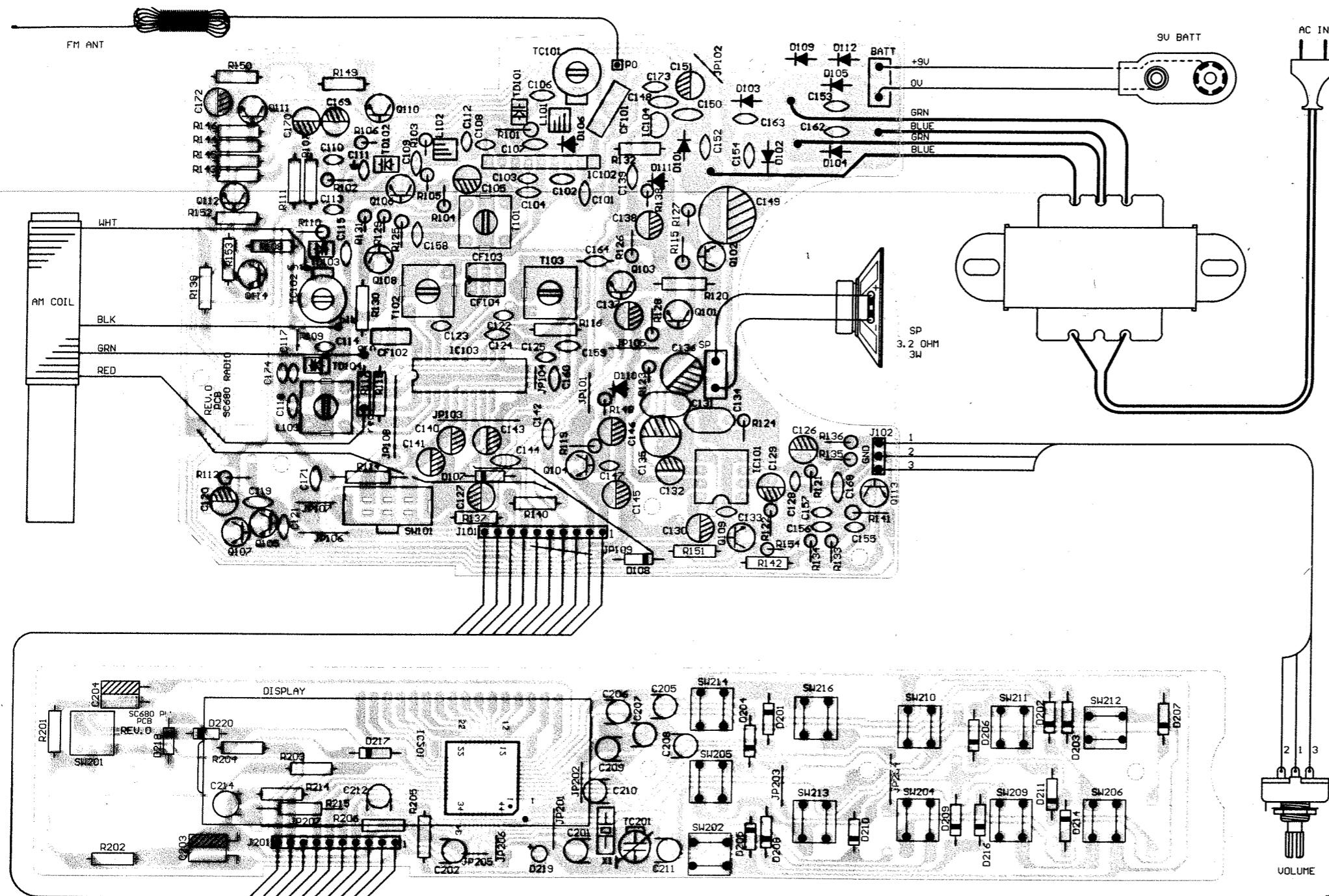
Druckplattenabbildungen Illustration of Printed Boards
